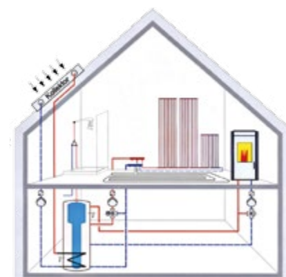
Heizwärme- und Warmwassererzeugung durch Solarthermie und Kaminofen mit Wärmetauscher. © Sonnenhaus Institut e.V.
